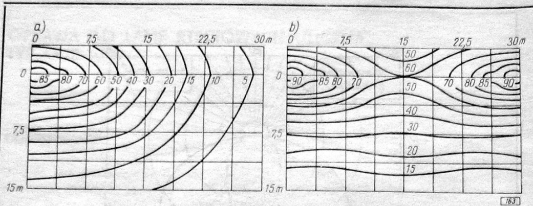
Krzywe izoluksów przy wysokości zawieszenia oprawy h=12\text{ m} , \delta=0^\circ a) dla jednej oprawy, b) dla dwóch opraw
