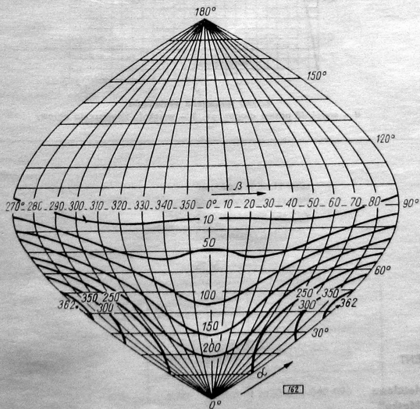
Krzywe izokandeli
