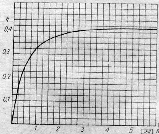
Krzywa sprawności oświetlenia d – szerokość pasma drogowego, h – wysokość zawieszenia oprawy
